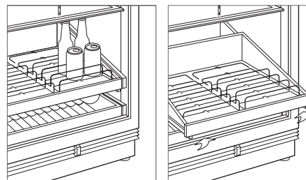
Clayette à boissons verticales
