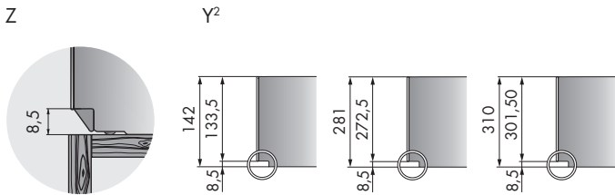
Dettaglio dimensioni cassetti
