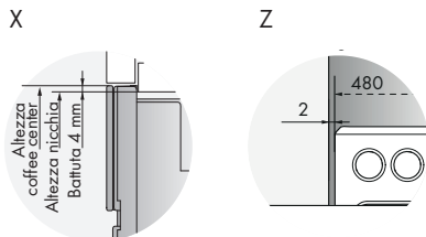
Dettaglio dimensioni Coffee-Center
