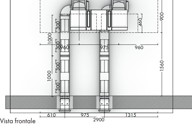
Vista frontale
