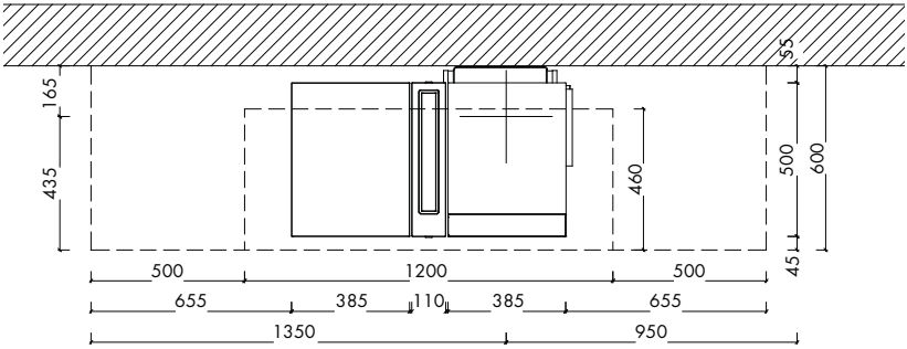
Pianta
