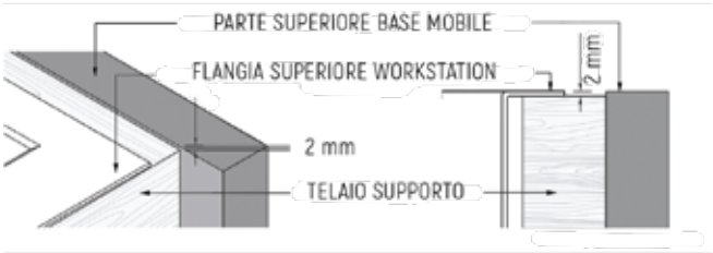
Dettaglio sezione A
