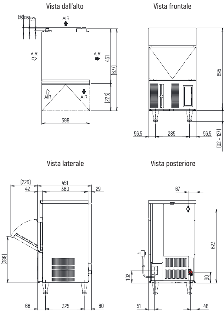
Dimensioni in mm
