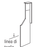
modifica deflettore parte inferiore
