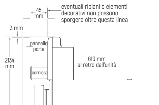
vista laterale bordo superiore (frigo e freezer a colonna)
