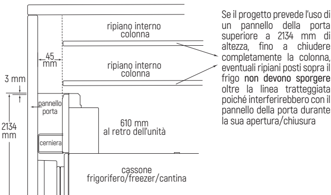
vista laterale bordo superiore
