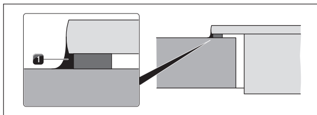
Fig. 5.18 Silicone per montaggio in battuta
