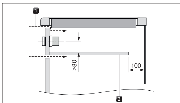
Fig. 5.7 Alimentazione aria sopra l'area frontale
