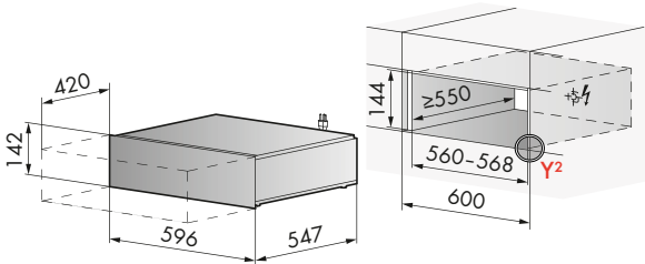
Installazione integrata con pannello cucina
