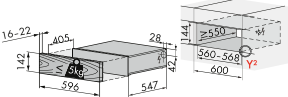
Installazione integrata con pannello cucina
