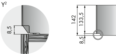
Dettaglio dimensioni lato frontale
