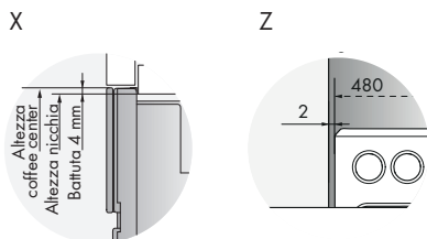
Dettaglio dimensioni Coffee-Center
