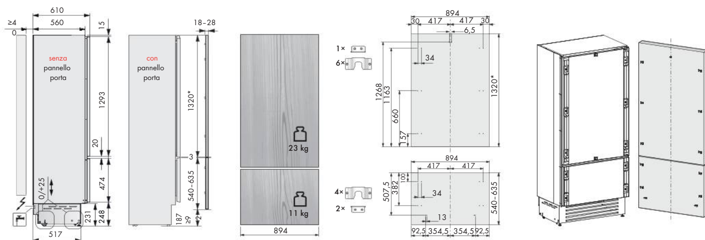
Vista assonometrica dettaglio fori pannelli
