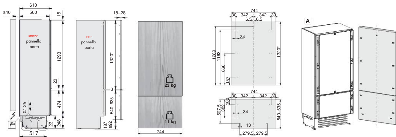
Vista assonometrica dettaglio fori pannelli
