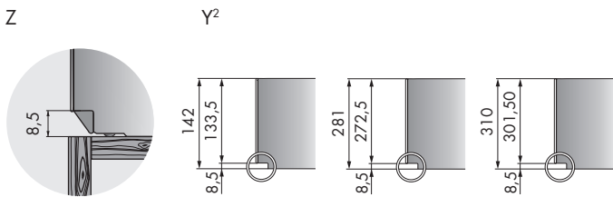
Dettaglio dimensioni cassetti
