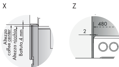
Dettaglio dimensioni Coffee-Center
