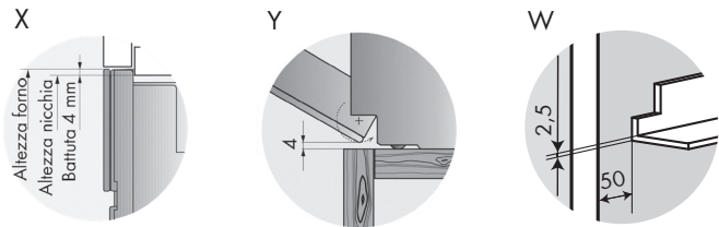
Dettaglio dimensioni forni
