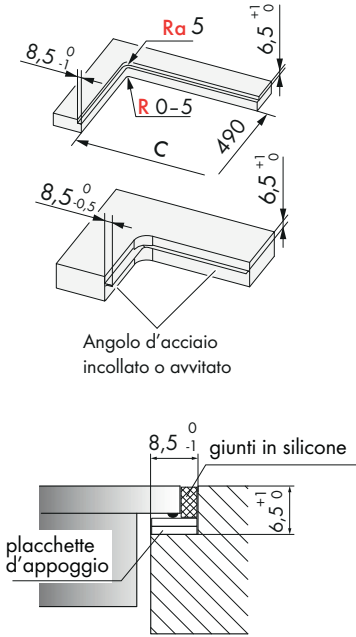
Dettaglio Z
