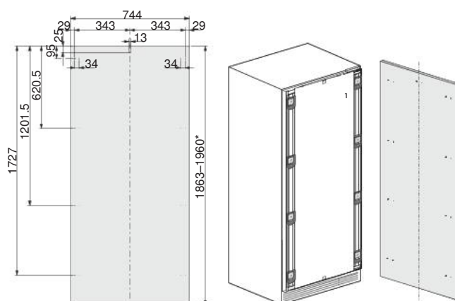
Vista assometrica dettaglio fori pannelli
