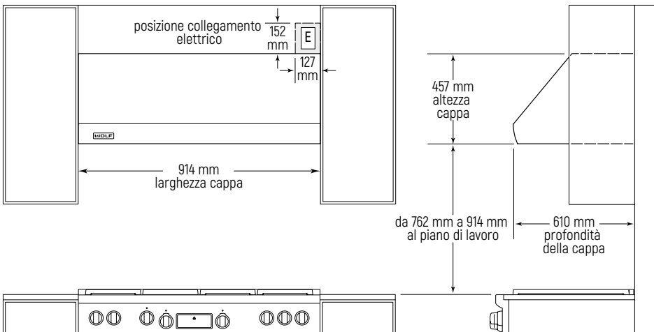
vista frontale
