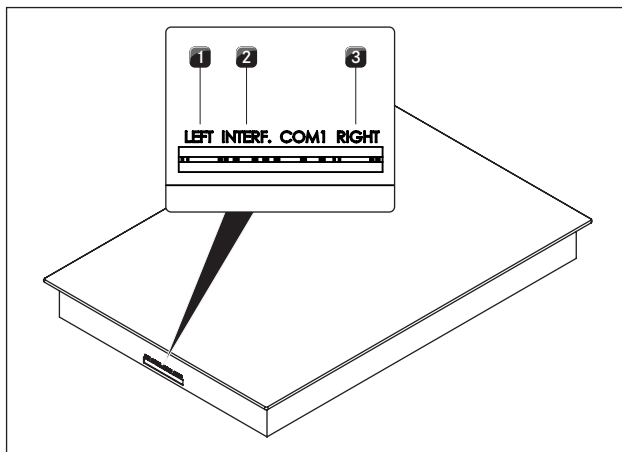
Fig. 5.23 Collegamento manopola di comando sul lato anteriore del piano cottura
