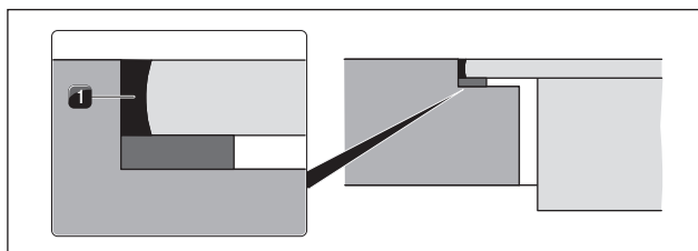
Fig. 5.20 Sigillante in silicone per montaggio a filo piano
