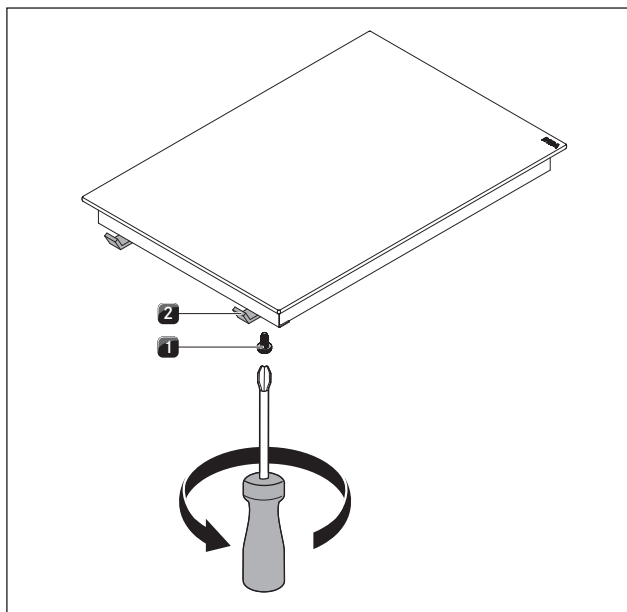
Fig. 5.19 Staffe di fissaggio
