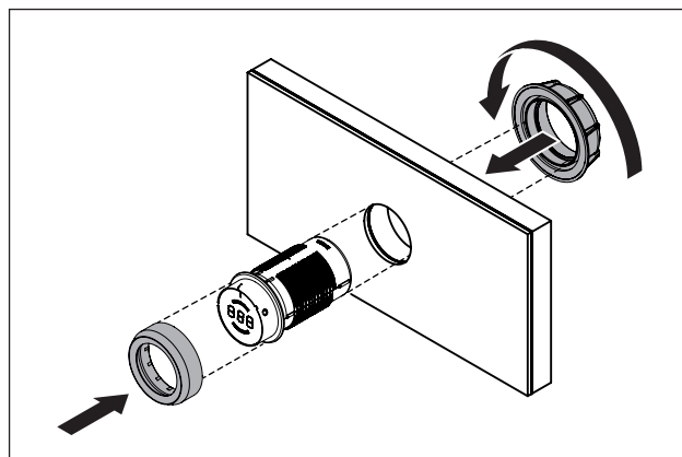
Fig. 5.14 Montaggio manopola di comando
