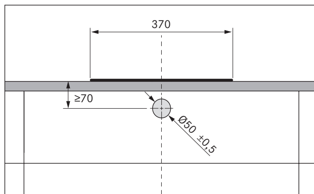
Fig. 5.13 Schema di foratura
