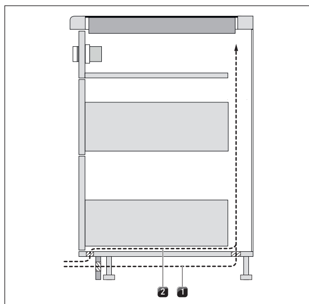
Fig. 5.9 Alimentazione aria attraverso l'area dello zoccolo
