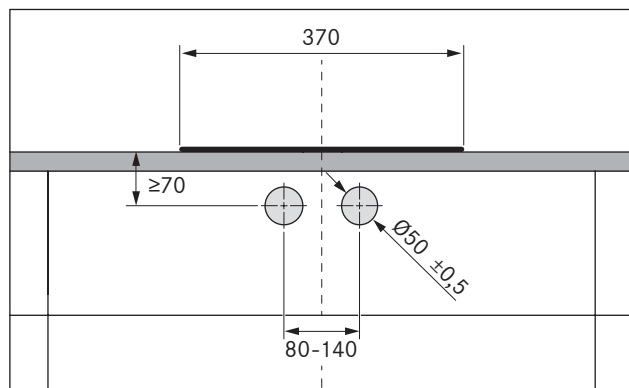
Fig. 5.11 Schema di foratura
