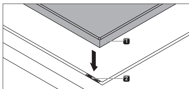
Fig. 5.18 Piano di cottura e pannelli di compensazione altezza
