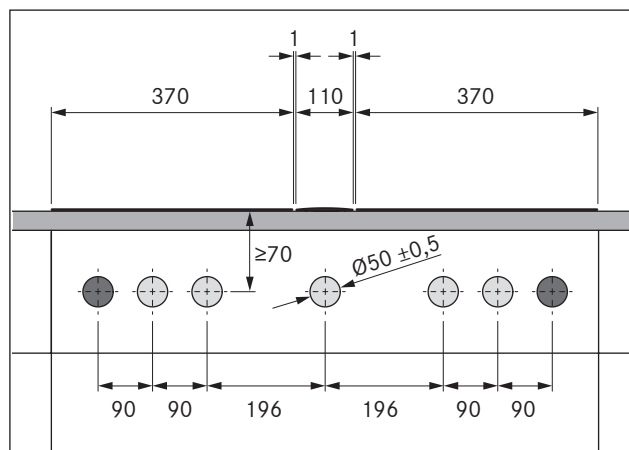
Fig. 5.15 Forature per pannelli di copertura con 2 piani cottura e 1 aspiratore
