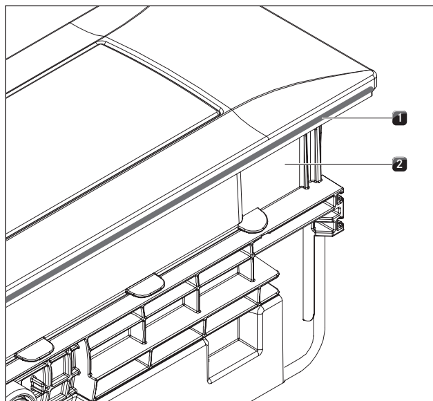
Fig. 5.7 Rimuovere il profilo di plastica laterale sull'aspiratore per piano cottura
