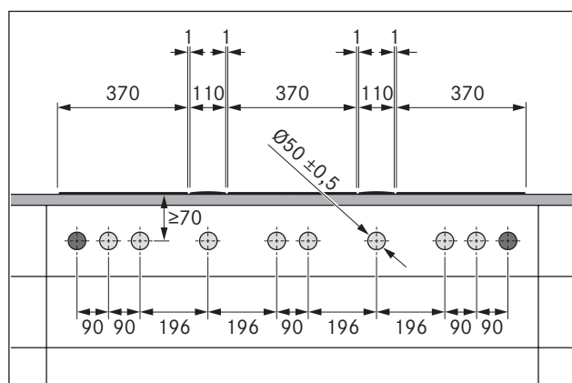
Fig. 5.16 Forature pannello di copertura per 3 piani cottura e 2 aspiratori
